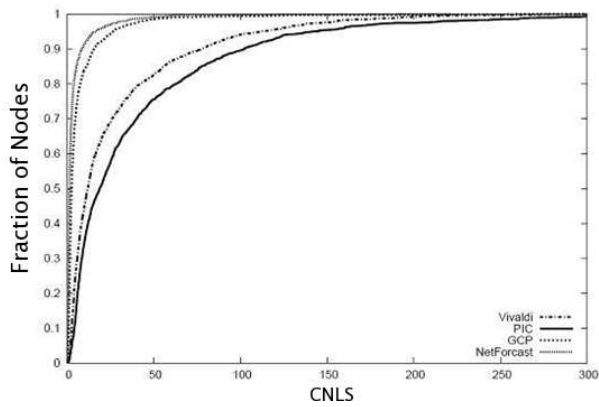
Fig. 3. CNLS distribution
